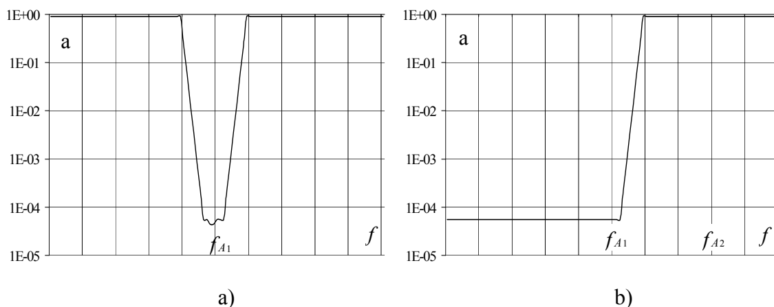
Figura 6.2 Caracteristica filtrului de rejectare a fundamentalei în cazul: a) FOB; b) FTS
