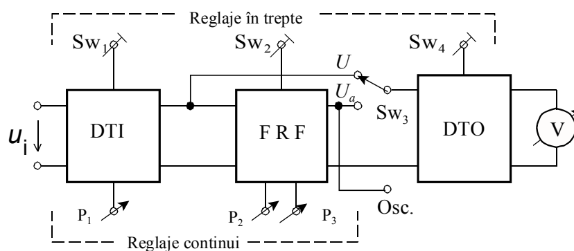
Figura 6.1 Distorsiometrul: schema bloc simplificată.
