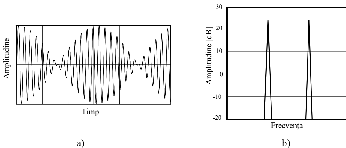
Figura 6.6 Semnalul de test a distorsiunilor de intermodulație vizualizat cu: a) osciloscopul; b) analizorul de spectru.
