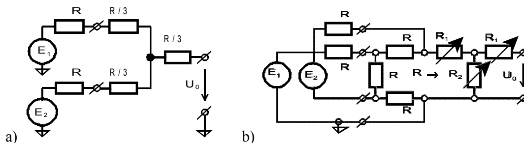
Figura 6.5 Obținerea semnalului de testare a distorsiunilor de intermodulație prin sumare cu rețea rezistivă: a) în stea; b) în punte.
