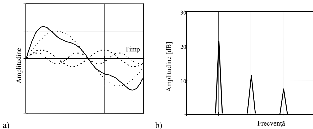
Figura 6.3 Reprezentarea unui semnal distorsionat în domeniul: a) timp; b) frecvență.
