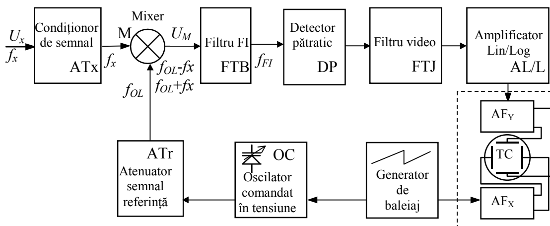
Figura 6.4 Analizorul de spectru superheterodină cu simplă schimbare de frecvență.
