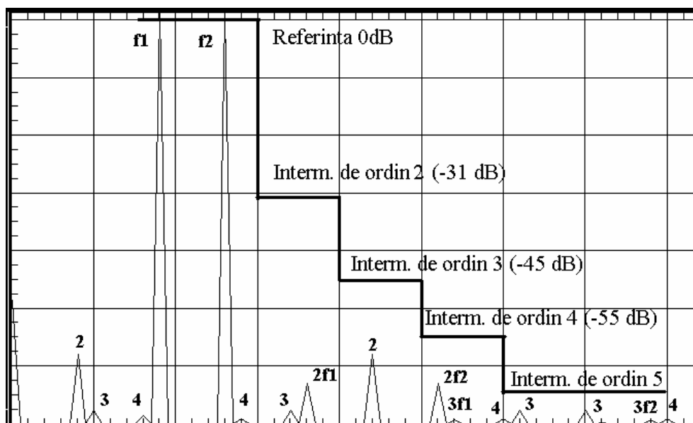
Figura 6.7 Imaginea rezultată pe ecranul analizorului de spectru la testarea liniarității unui diport cu două tonuri de f_1 = 900 și f_2 = 1300 Hz.
