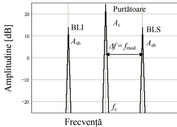
Figura 6.8 Imagine pe ecranul analizorului de spectru la măsurarea gradului de modulație în amplitudine ( m = 60\% ): BLI = banda laterală inferioară; BLS = banda laterală superioară.
